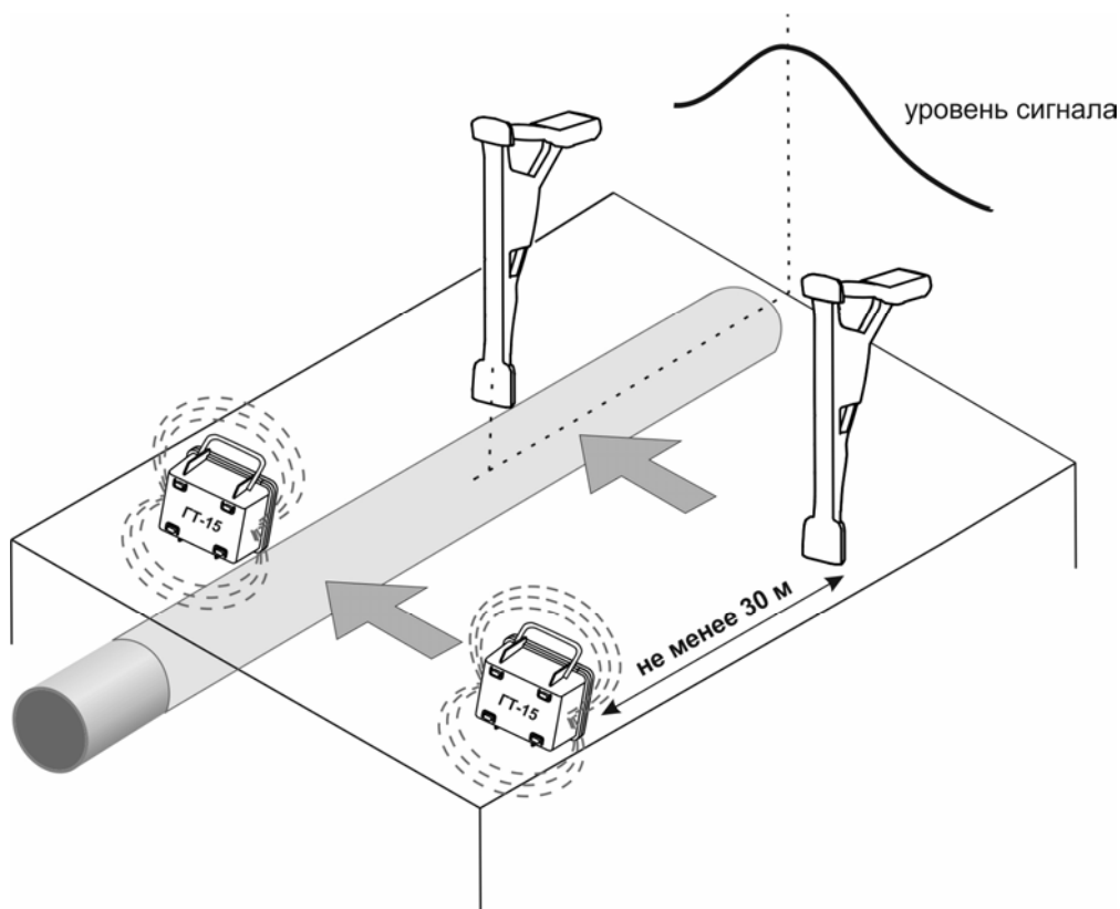
Рисунок 4.4.2.2 – Обследование участков местности с помощью ГТ-15
