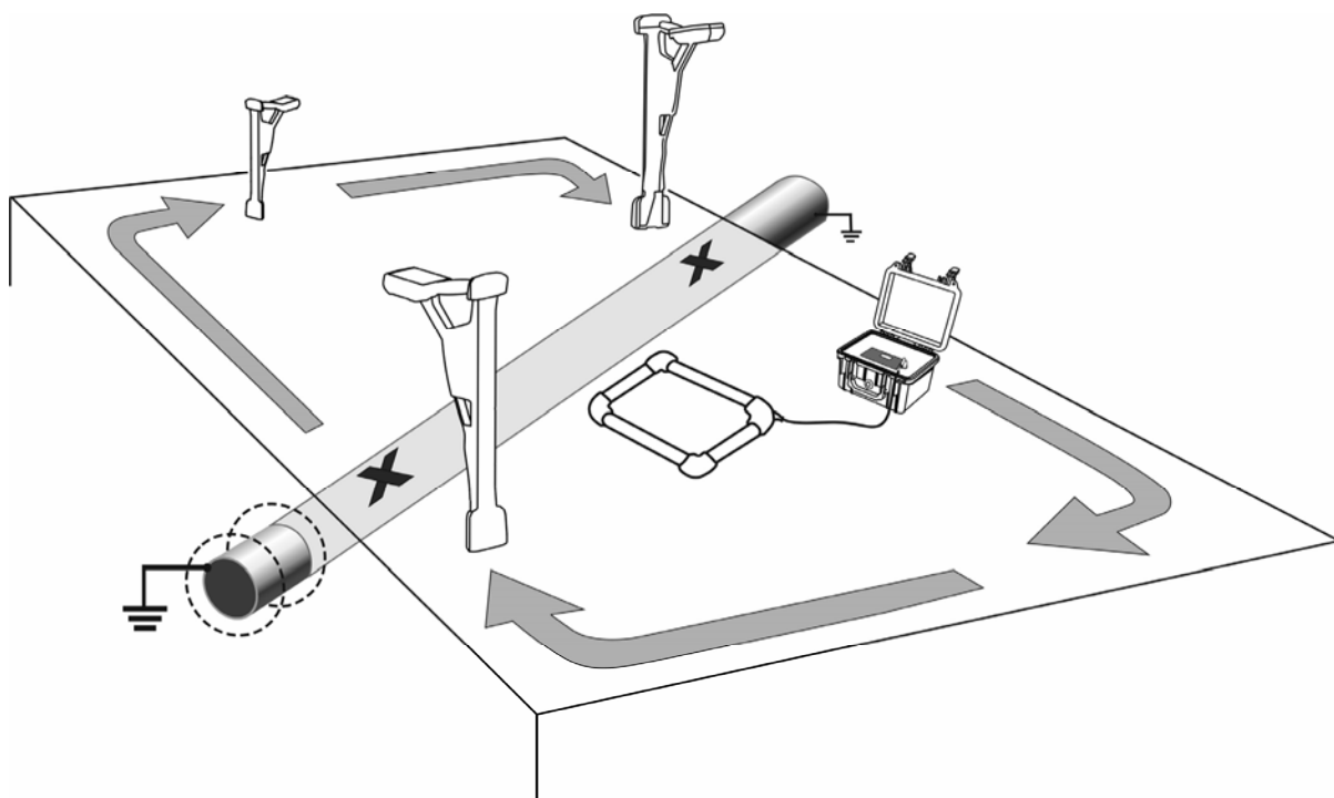
Рисунок 4.4.2.1 – Обследование участков местности с использованием рамки РП-02
