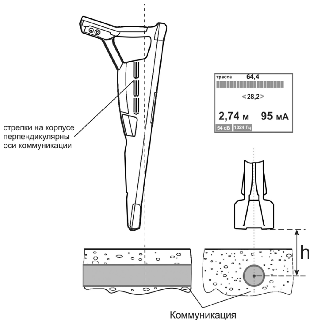
Рисунок 4.3 – Показания глубины залегания и тока
