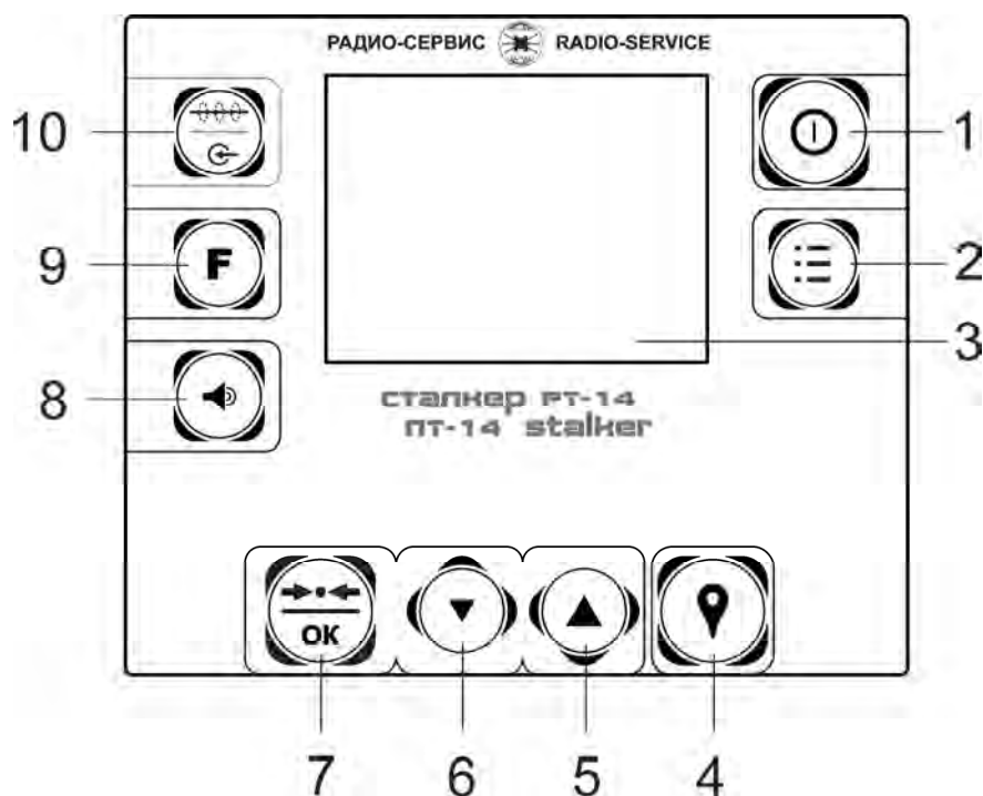
Рисунок 1.4.2 - Передняя панель приёмника
