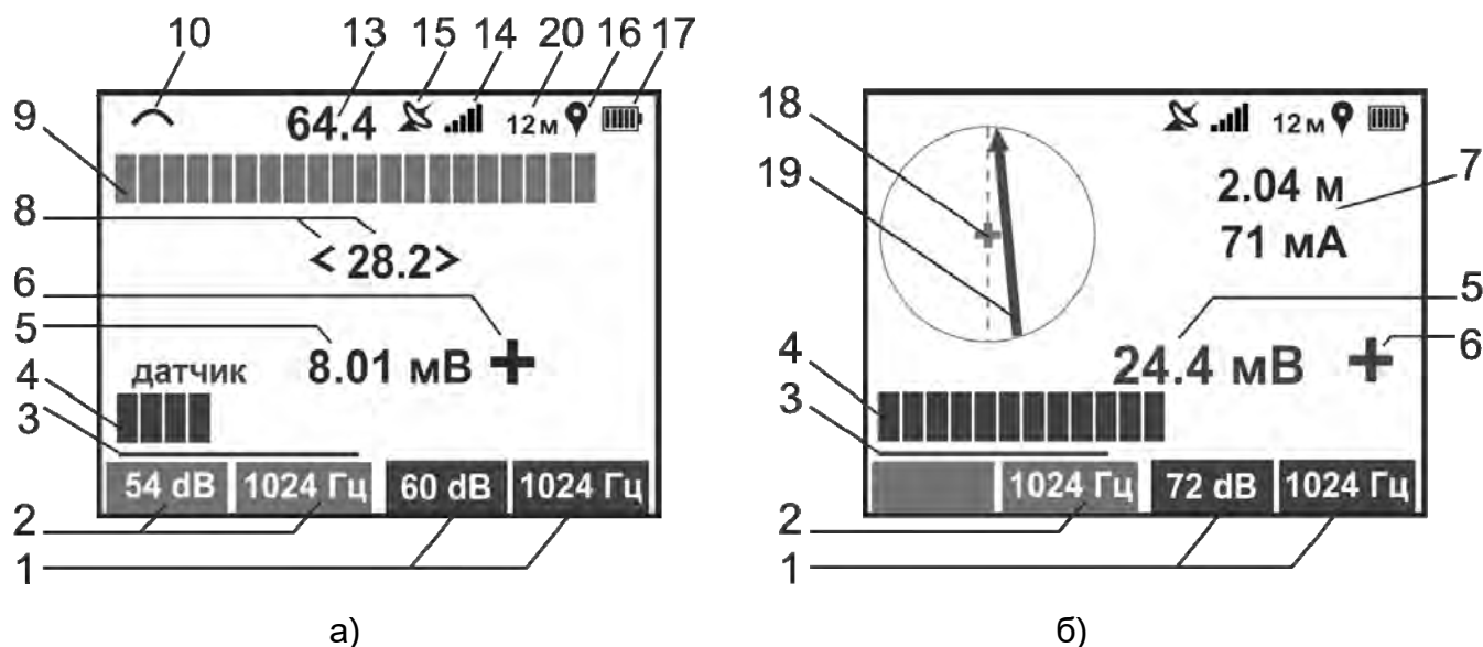
Рисунок 3.3 – Индикация приемника в режиме «ТРАССА-ДАТЧИК»
