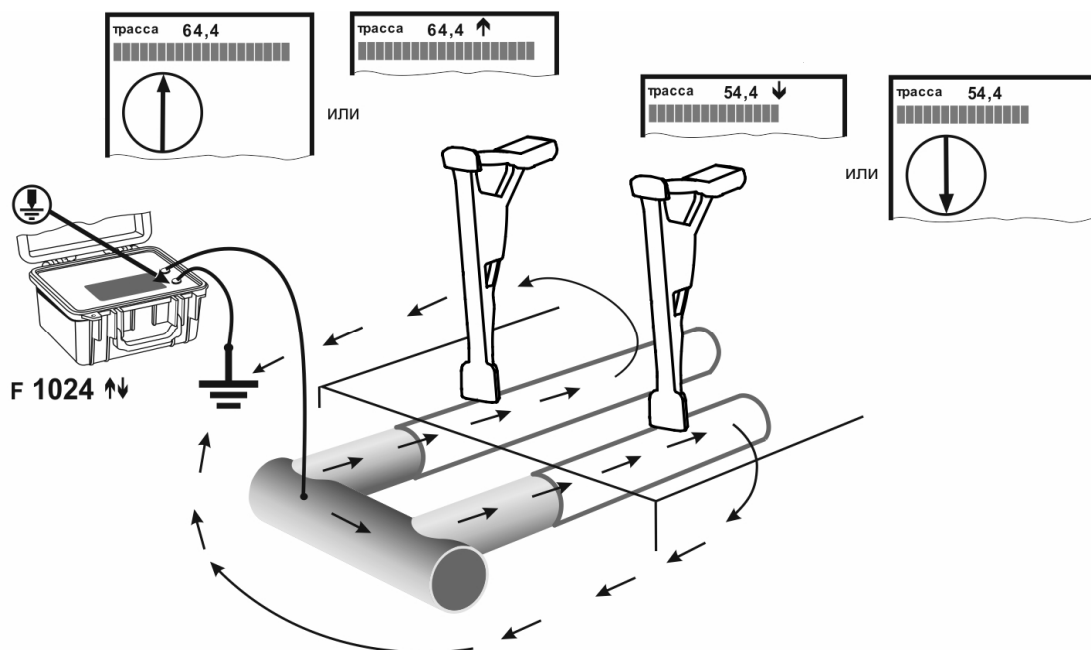
Рисунок 4.2.4.2 – Направление тока и показания приемника при гальванически связанных коммуникациях
