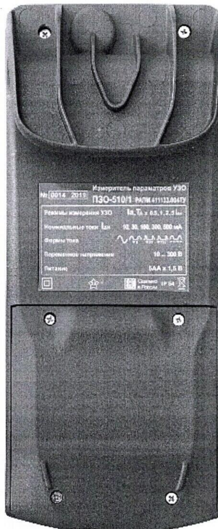
Рисунок 4 – Общий вид измерителей параметров УЗО ПЗО-510/1. Вид сзади
