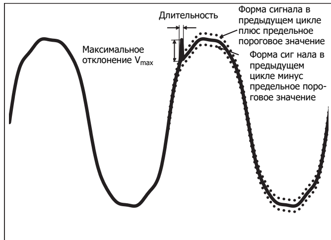
Рисунок 14. Отклонение формы сигнала
