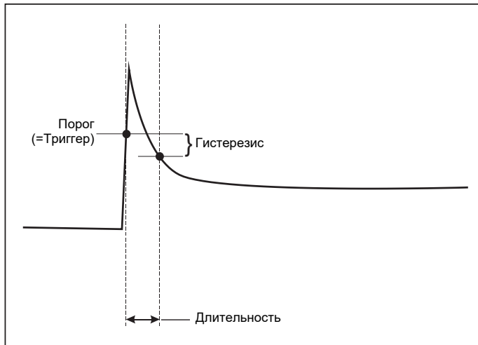
Рисунок 15. Пусковые характеристики
