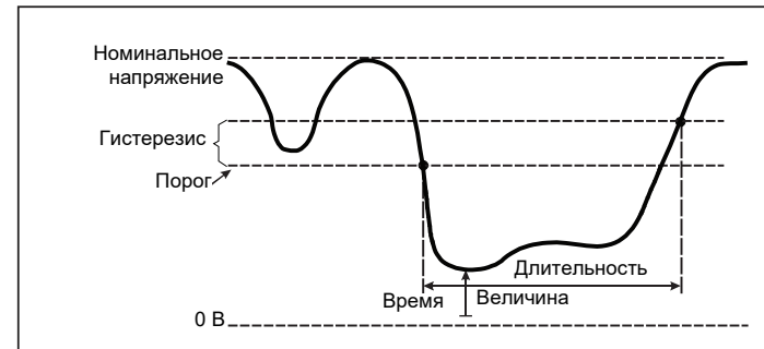
Рисунок 12. Характеристики прерывания напряжения
