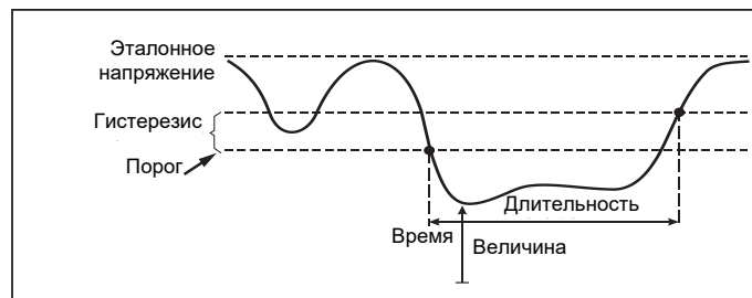
Рисунок 10. Характеристики кратковременного понижения напряжения
