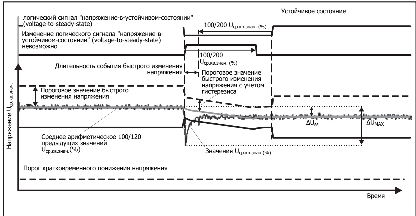
Рисунок 13. Характеристики быстрого изменения напряжения
