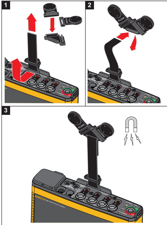
Рисунок 2. Комплект магнитной подвески
