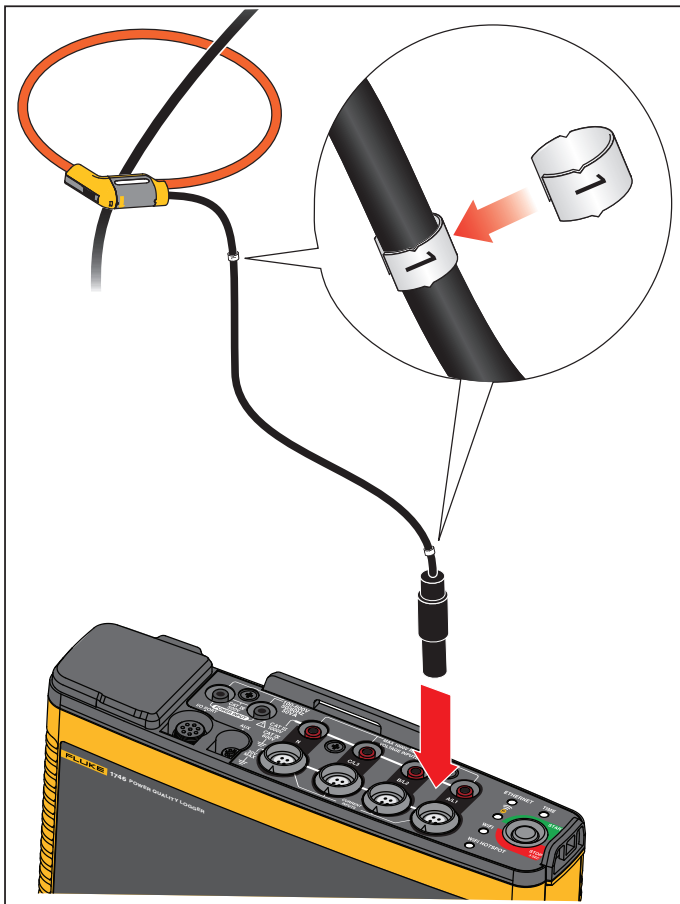
Рисунок 4. Измерительные провода с цветовой кодировкой
