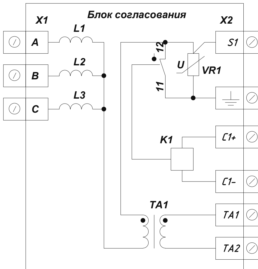
Рисунок Б.2 – Схема блока согласования
