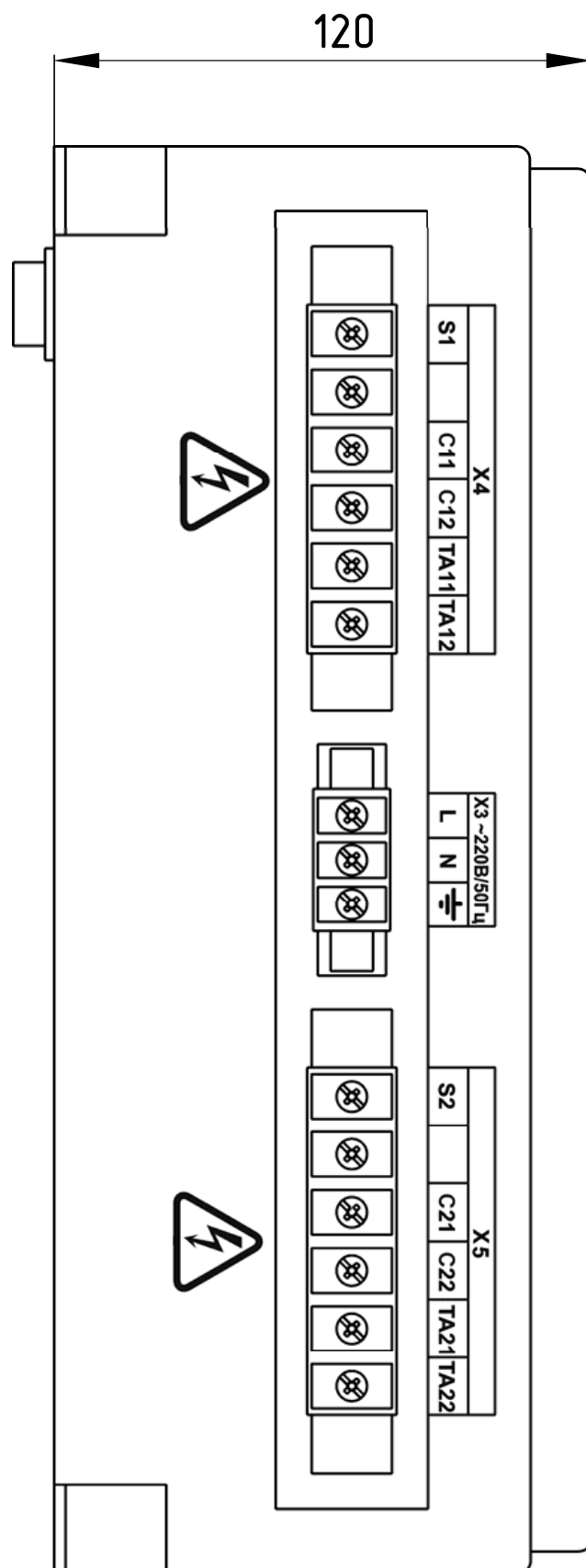
Рисунок А.1 – Внешний вид генератора. Боковая панель.
