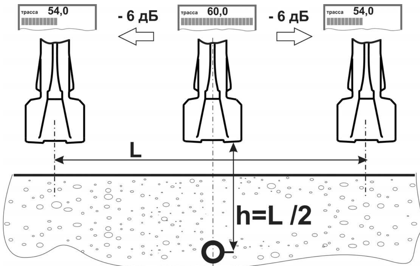
Рисунок 4.3.1 – Определение глубины залегания методом «-6дБ»
