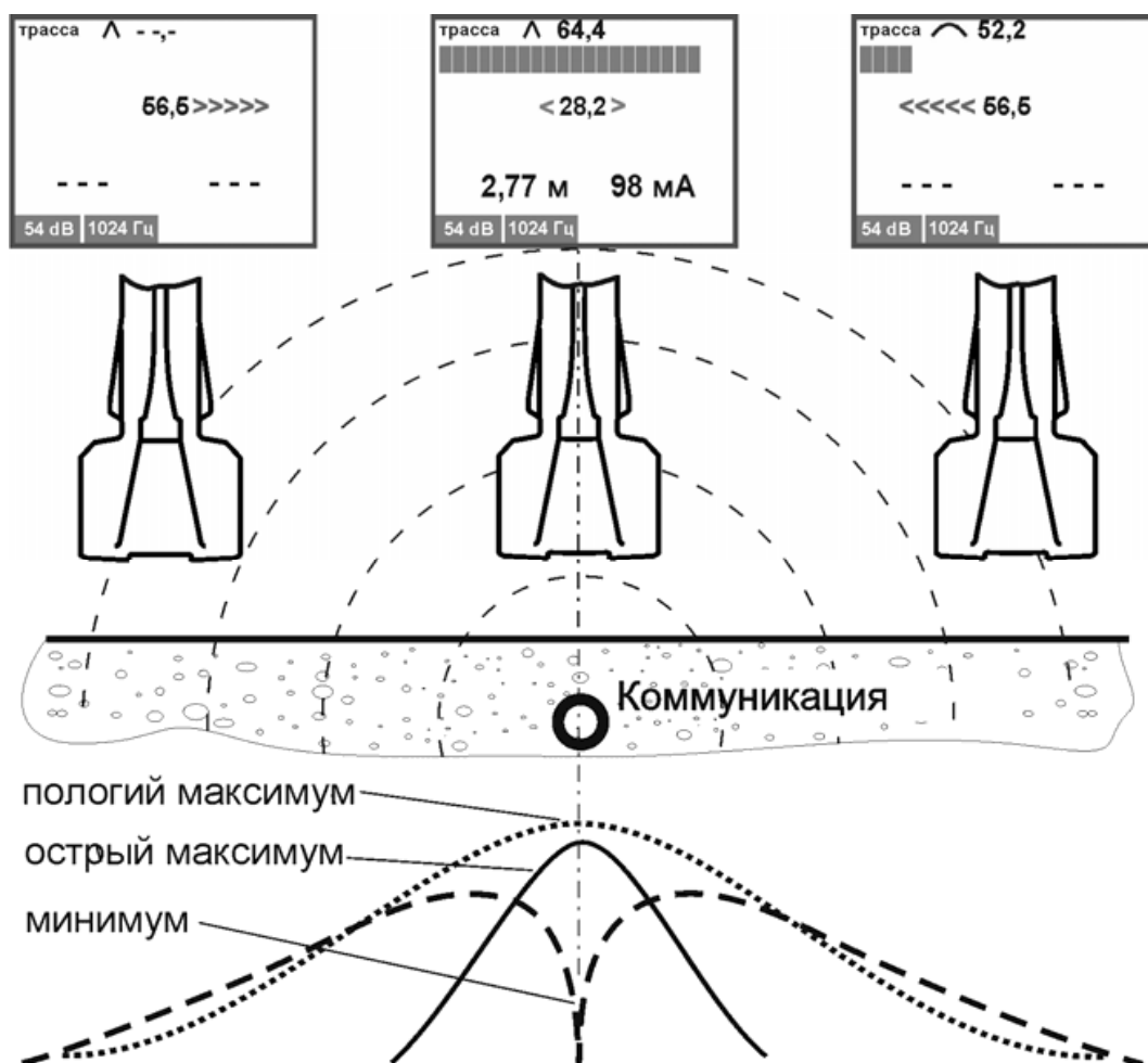
Рисунок 4.2.1 – Изменение уровней сигналов при смещении приёмника относительно оси коммуникации
