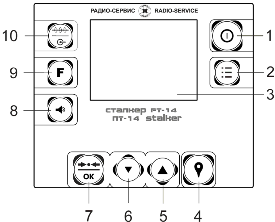
Рисунок 1.4.2 – Передняя панель приёмника
