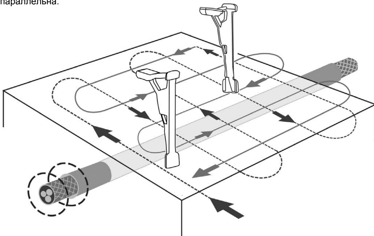
Рисунок 4.4.1 – Обследование участков местности без генератора
