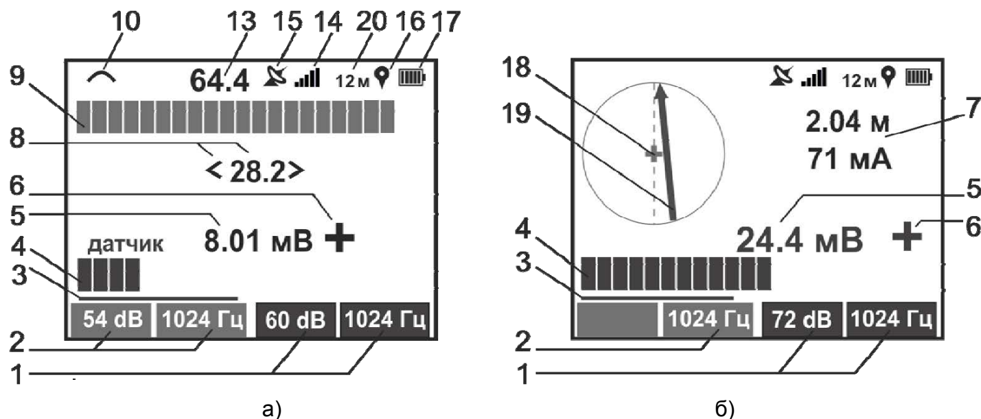
Рисунок 3.3 – Индикация приемника в режиме «ТРАССА-ДАТЧИК»
