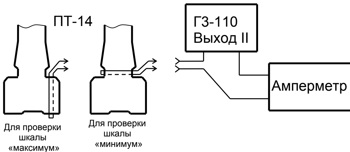
Рисунок 13.5.3 – Схема рабочего места для проверки чувствительности
