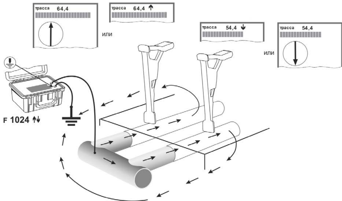
Рисунок 4.2.4.2 – Направление тока и показания приемника при гальванически связанных коммуникациях
