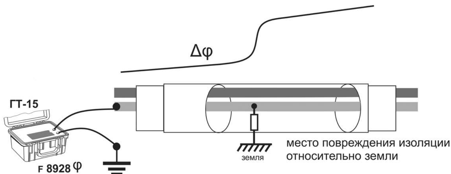
Рисунок 5.3.3.2 – Схема подключения и сдвиг фазы при поиске повреждения изоляции фазовым методом
