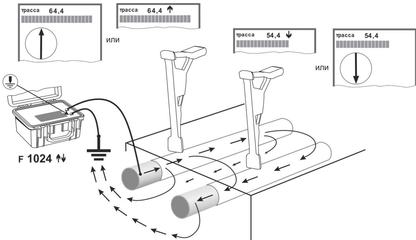
Рисунок 4.2.4.1 – Направление тока и показания приемника при гальванически несвязанных коммуникациях
