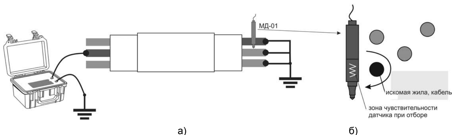
Рисунок 5.4.1 – Схема подключения при отборе жил кабеля
