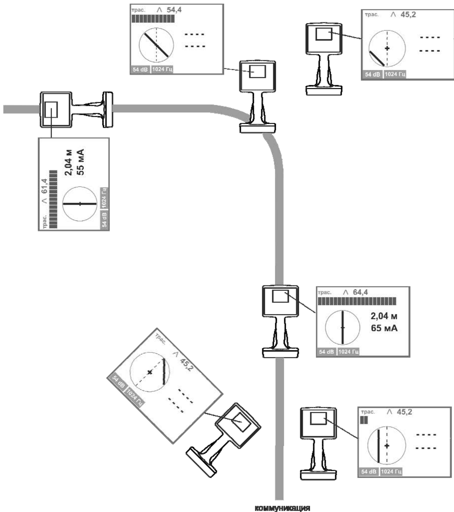
Рисунок 4.2.3 – Поиск с включенной функцией «КОМПАС»
