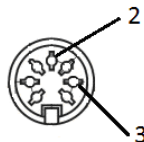
Рисунок 13.5.4 – Нумерация контактов гнезда «ДАТЧИК»
