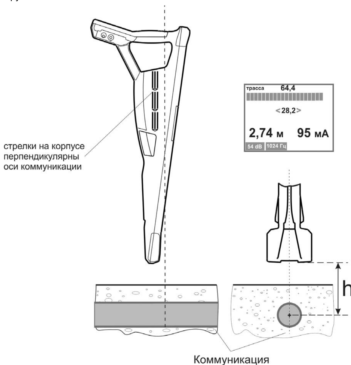
Рисунок 4.3 – Показания глубины залегания и тока
