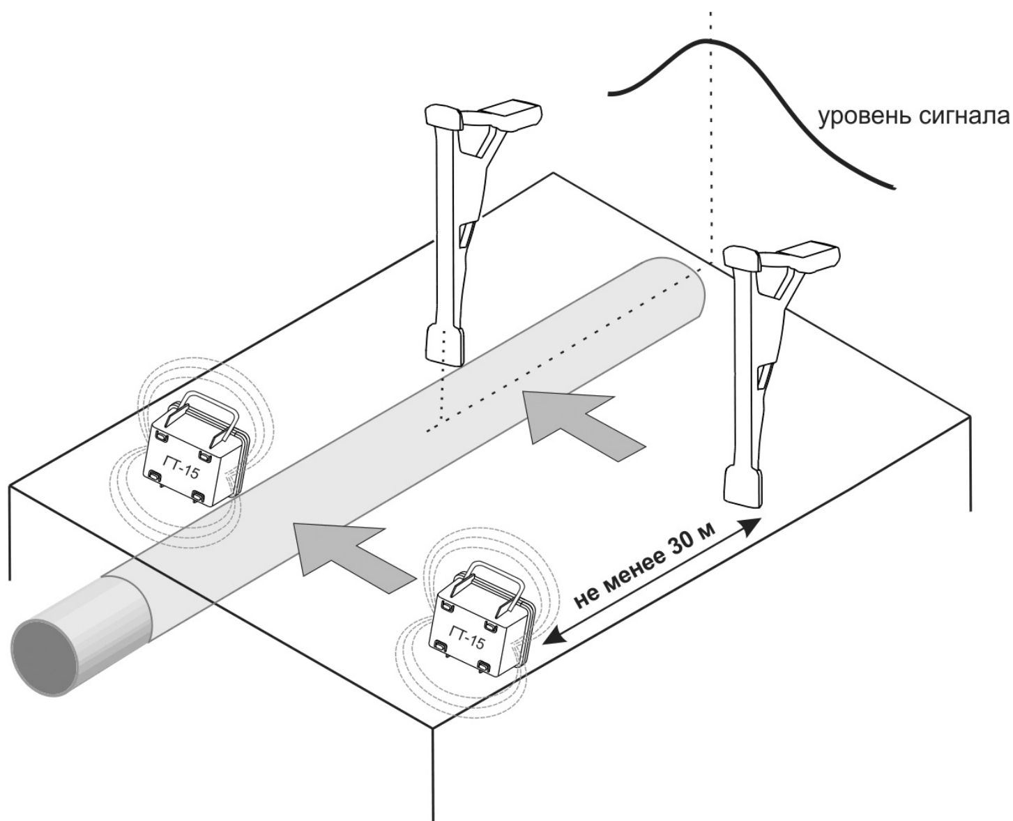
Рисунок 4.4.2.2 – Обследование участков местности с помощью ГТ-15
