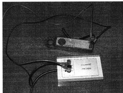
Рисунок 7 – Комплект измерения тока с токовыми клещами ТК-200DC «/200DC»
