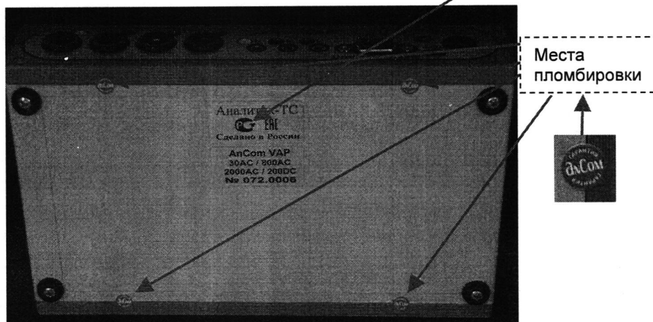
Рисунок 3 – Места пломбировки и нанесения знака утверждения типа на корпусе приборного блока
