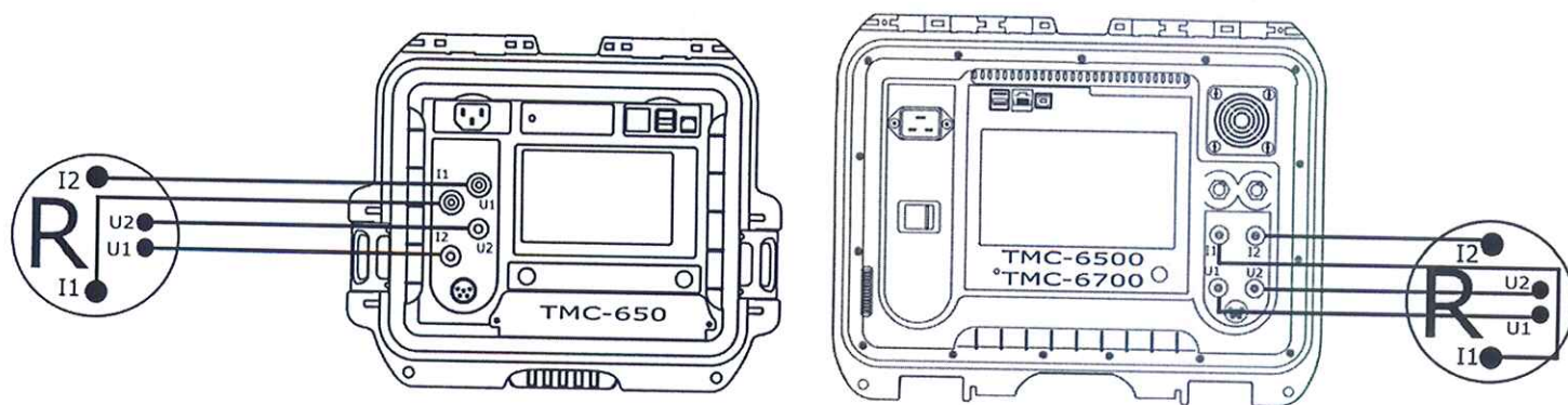
Рисунок 1 - Структурная схема определения основной абсолютной погрешности измерения электрическому сопротивлению постоянному току до 10 А.
