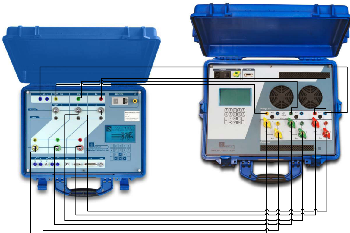
Рисунок А.3 - Схема соединения генератора «Энергоформа-3.3-120М» и прибора «Энергомонитор-3.1КМ» при токе от 12 до 120 А.
