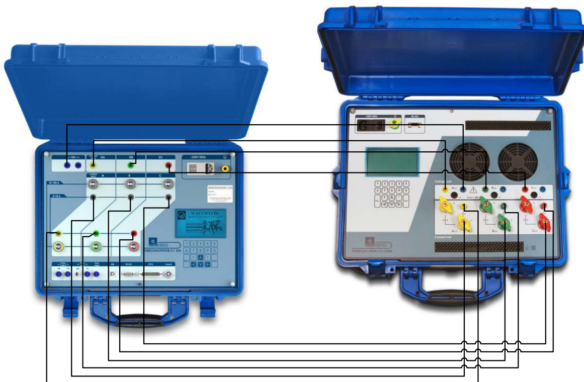
Рисунок А.2 - Схема соединения генератора «Энергоформа-3.3-120М» и прибора «Энергомонитор-3.1КМ» при токе до 12 А.
