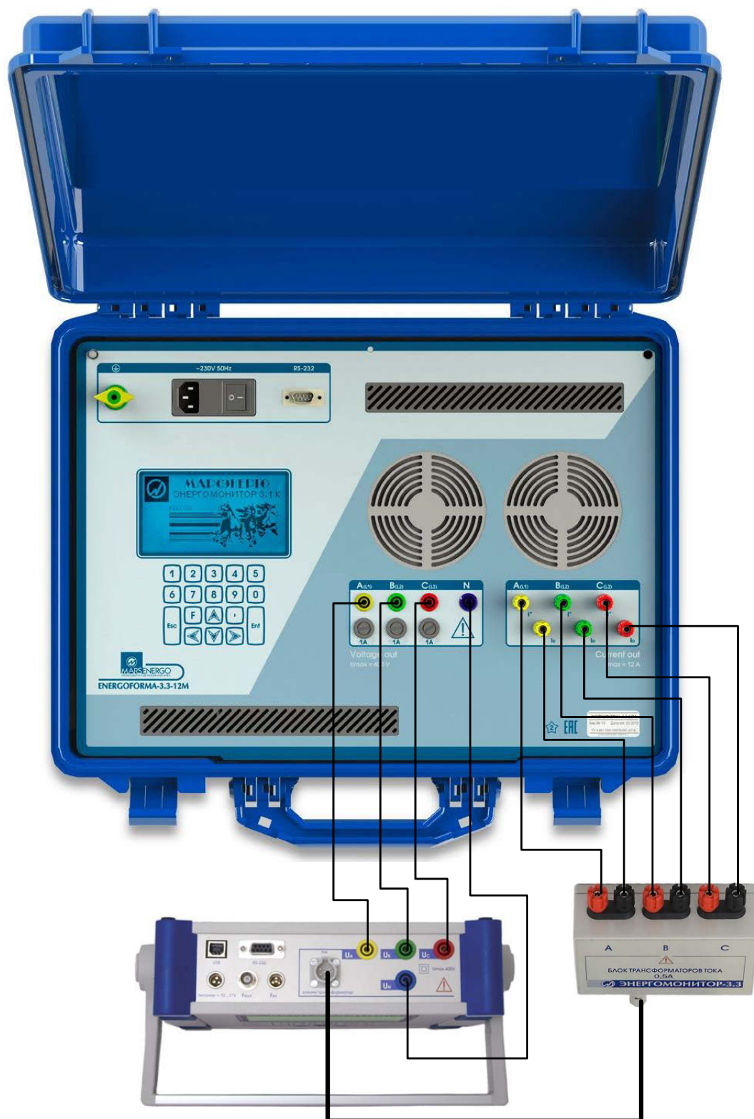
Рисунок А.1 - Схема соединения генератора «Энергоформа-3.3-12М» и прибора «Энергомонитор-3.3Т1»
