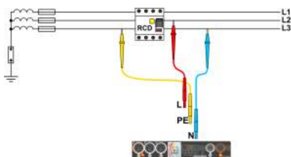
Рис. 4.2 Тестирование УЗО без участия провода PE
