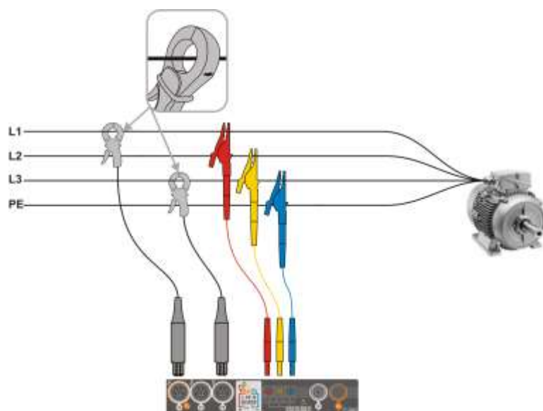
Рис. 6.8 Схема подключения – трехфазная цепь с тремя рабочими проводами (измерение токов методом Arona)
