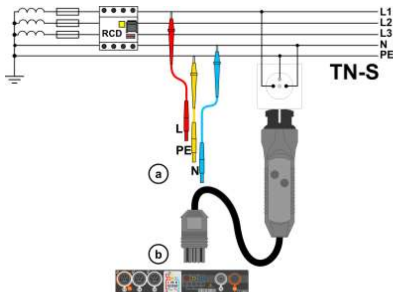
Рис. 3.3 Измерение в цепи TN-S
