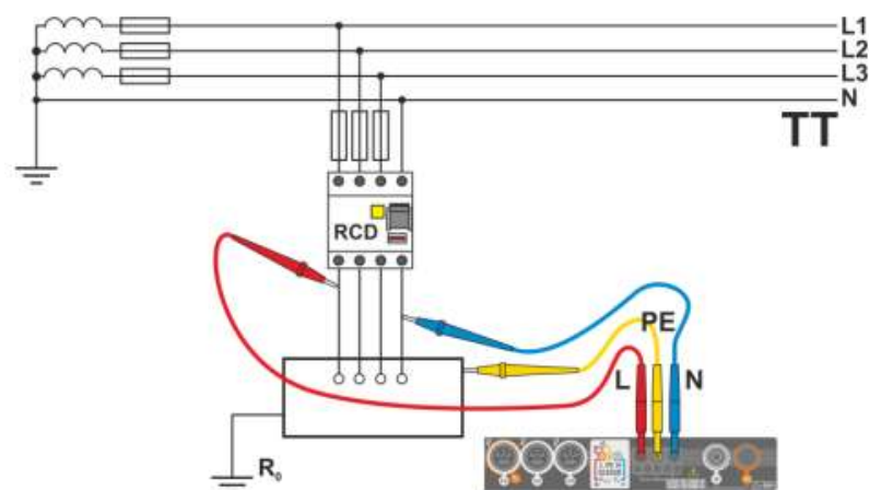
Рис. 3.4 Измерение в цепи TT
