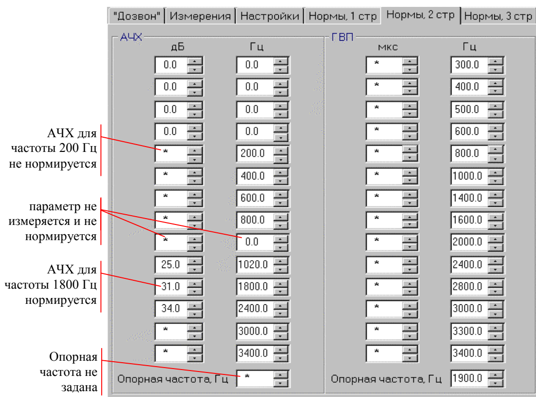
Рисунок 24. Нормы АЧХ / ГВП
