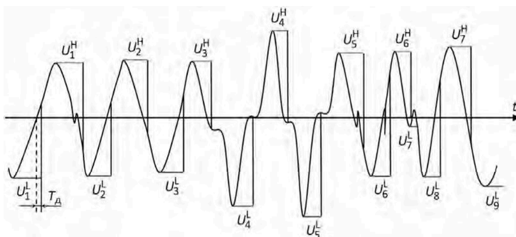
Рис. 4.57. Диаграмма работы прибора в режиме «СРЕДНЯЯ АМПЛИТУДА»:
