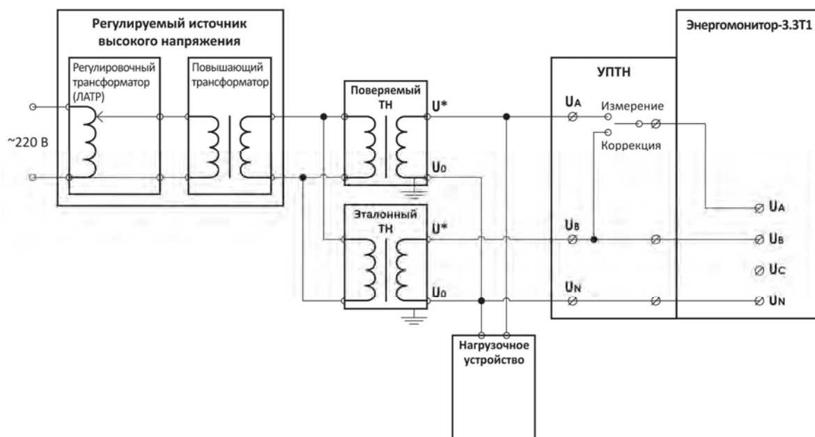
Рис. 4.30. Схема установки для поверки ТН
