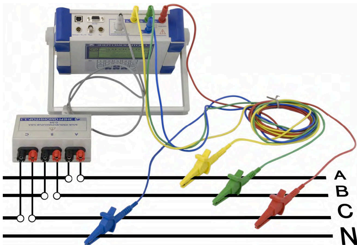
Рис. В.4. Схема подключения Прибора ЭМ-3.3Т1 к трехфазной четырехпроводной сети через БТТ
