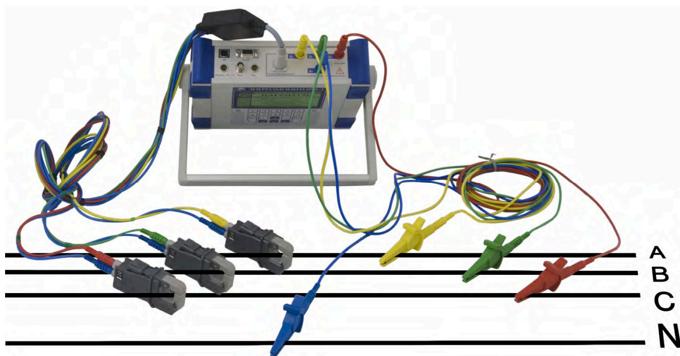
Рис. В.5. Схема подключения Прибора ЭМ-3.3Т1 к трехфазной четырехпроводной сети с помощью токоизмерительных клещей
