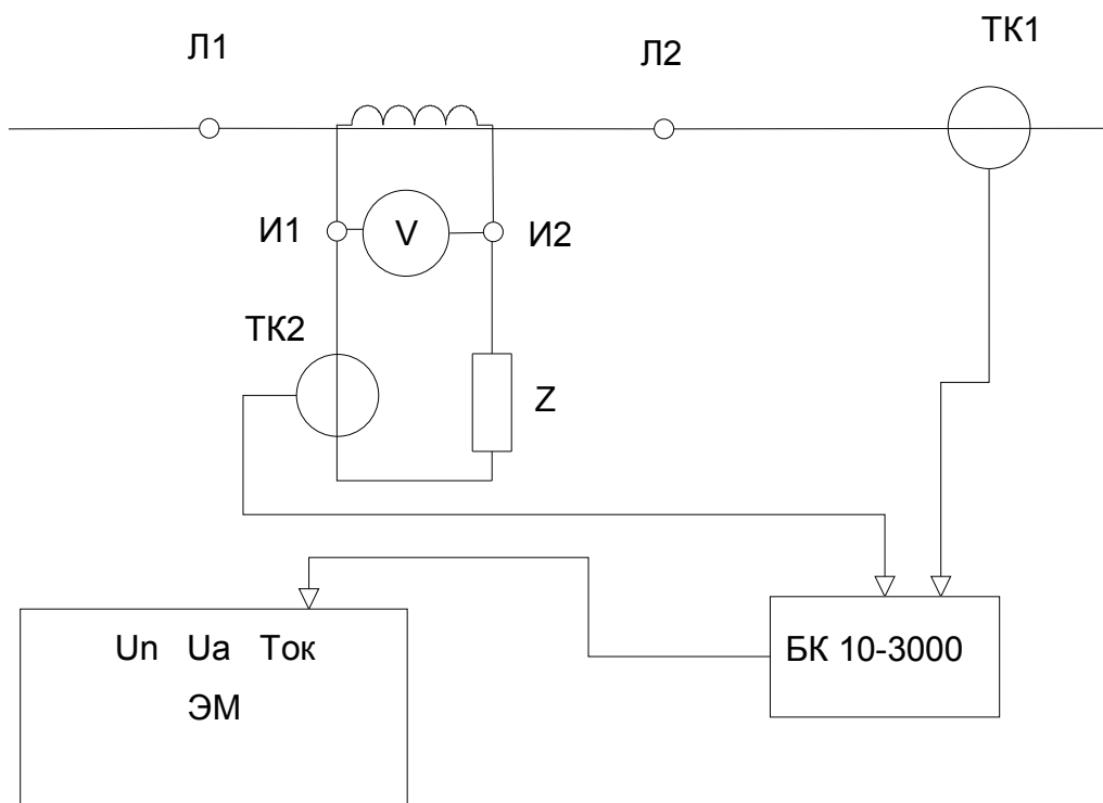
Рис. 4.466. Схема испытаний.
