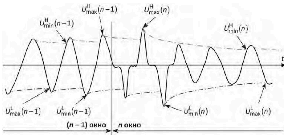
Рис. 4.54. Диаграмма работы прибора в режиме «АМПЛИТУДНЫЙ ДЕТЕКТОР»
