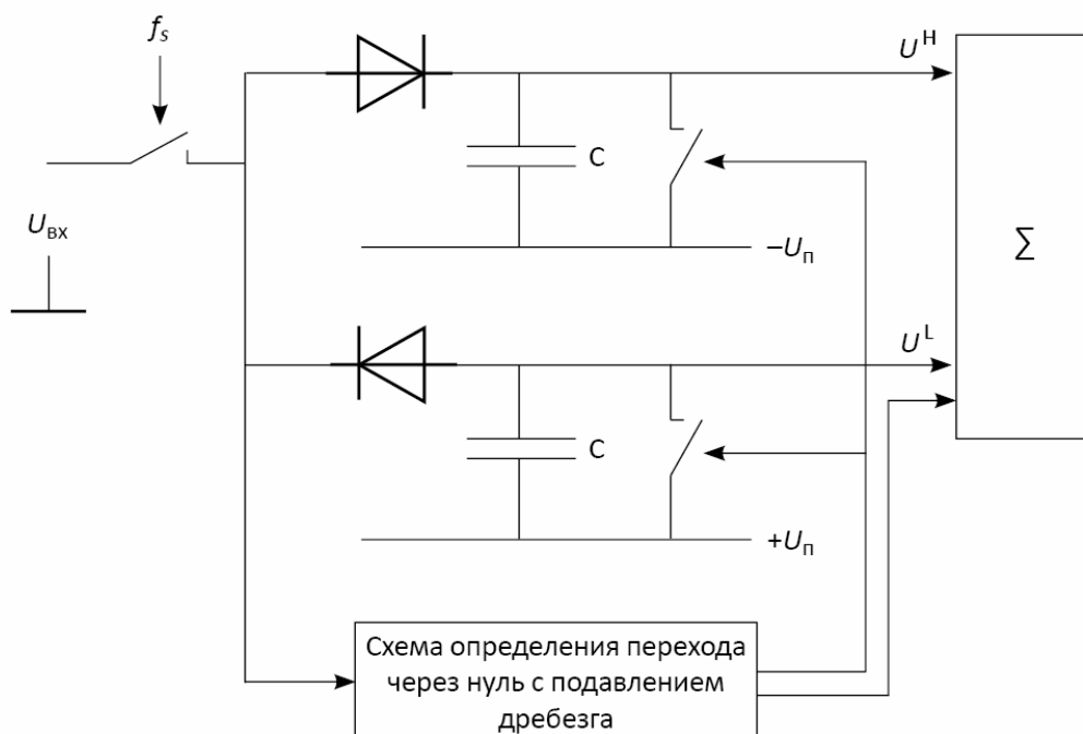
Рис. 4.56. Принцип обработки входного сигнала в режиме «СРЕДНЯЯ АМПЛИТУДА»:
