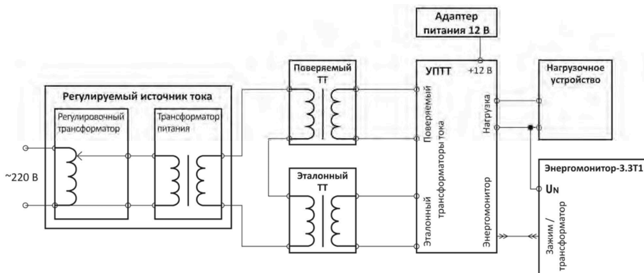
Рис. 4.38. Схема установки для поверки ТТ
