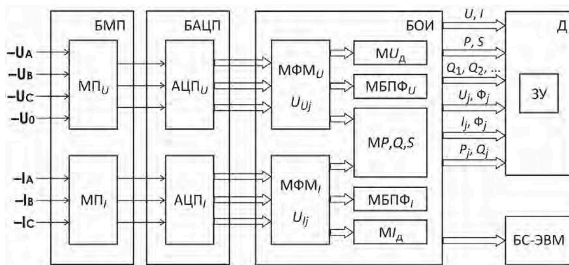
Рис. 2.1. Структурная схема Прибора ЭМ-3.3Т1:
