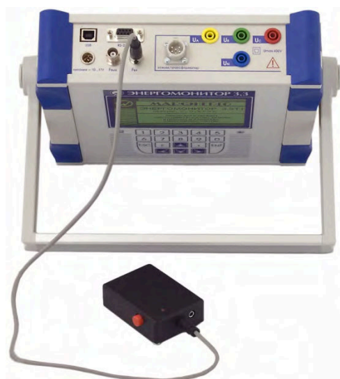
Рис. В.13. Схема подключения ПФИ к Прибору ЭМ-3.3Т1 при проверке индукционных и электронных (с оптическим импульсным выходом) счетчиков
