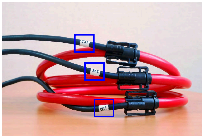
Рис. Б.12. Расположение маркировки «нагрузка» ➔ «генератор» на токоизмерительных клещах 300/3000 А
