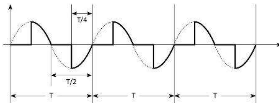
Рис. 2.19 - Форма выходного сигнала в режиме «Фазовое управление» (Т — период сигнала)
