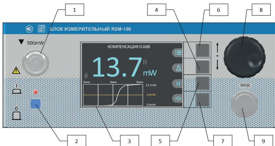
Рисунок 2. Передняя панель БИ
