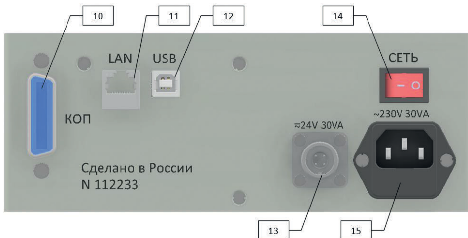
Рисунок 3. Задняя панель БИ
