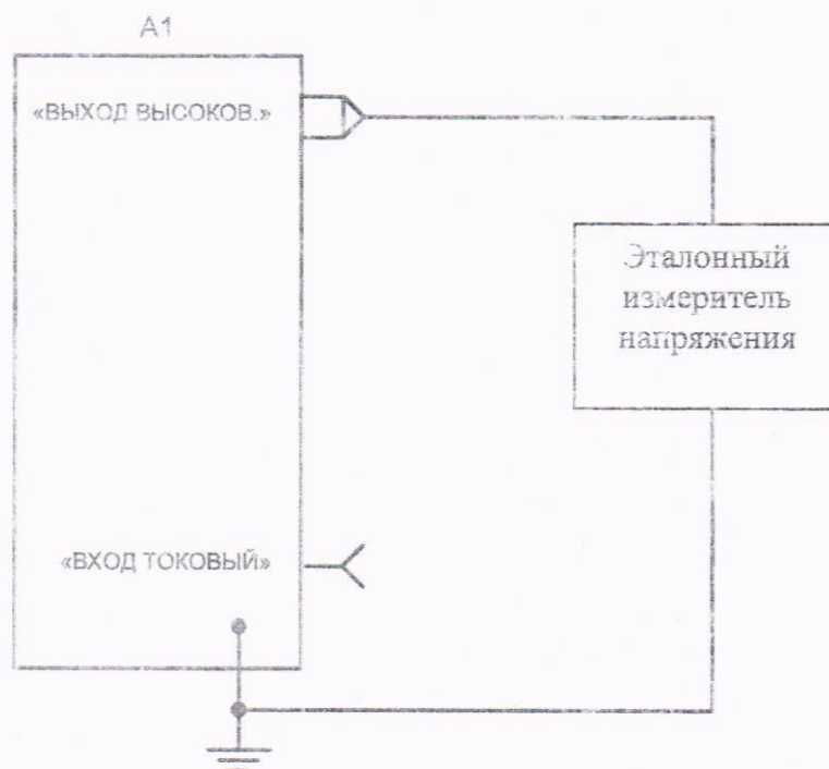
Рисунок 1 - Схема определения относительной основной погрешности измерений напряжения переменного тока промышленной частоты
