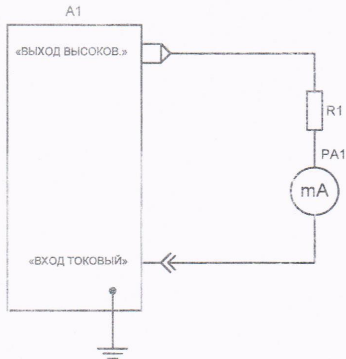
Рисунок 3 - Схема определения относительной погрешности измерений силы переменного тока промышленной частоты при незаземленной нагрузке
