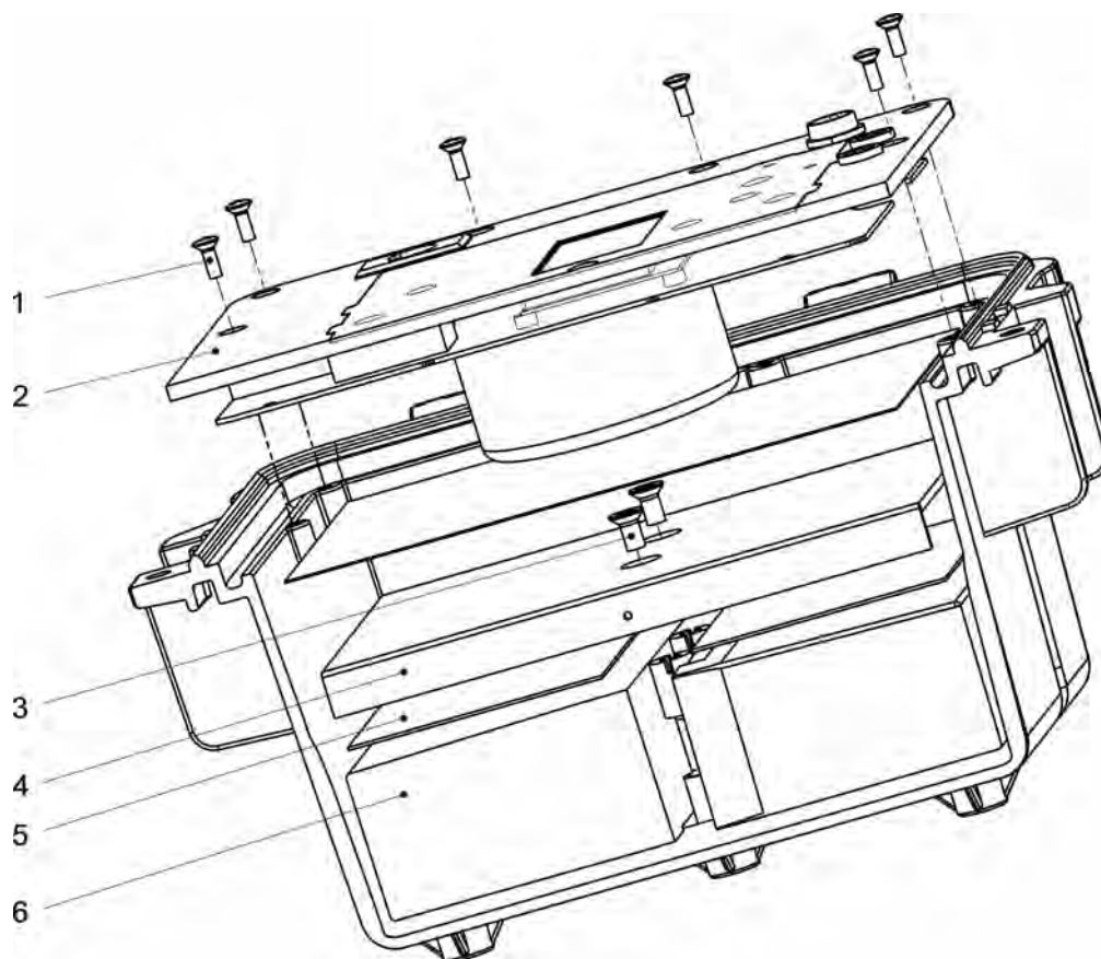
Рисунок 3.1 – Замена аккумуляторов
