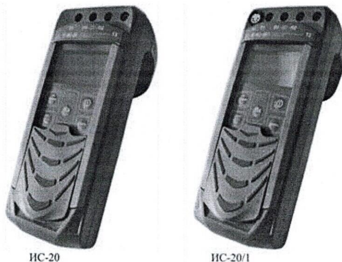
Рисунок 1 – Общий вид приборов ИС-20, ИС-20/1
