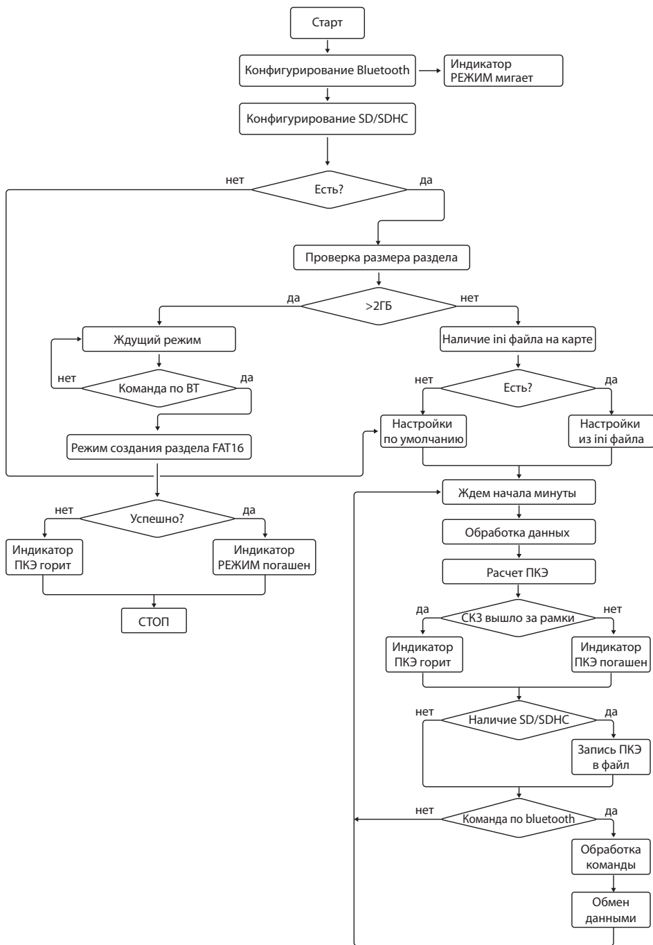
Рисунок 2. Алгоритм работы регистратора
