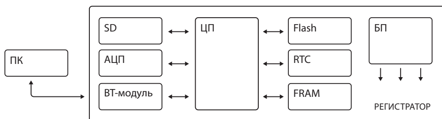
Рисунок 1. Структурная схема регистратора
