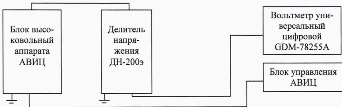
Рисунок 1 - Схема определения относительной основной погрешности измерений напряжения переменного тока промышленной частоты
