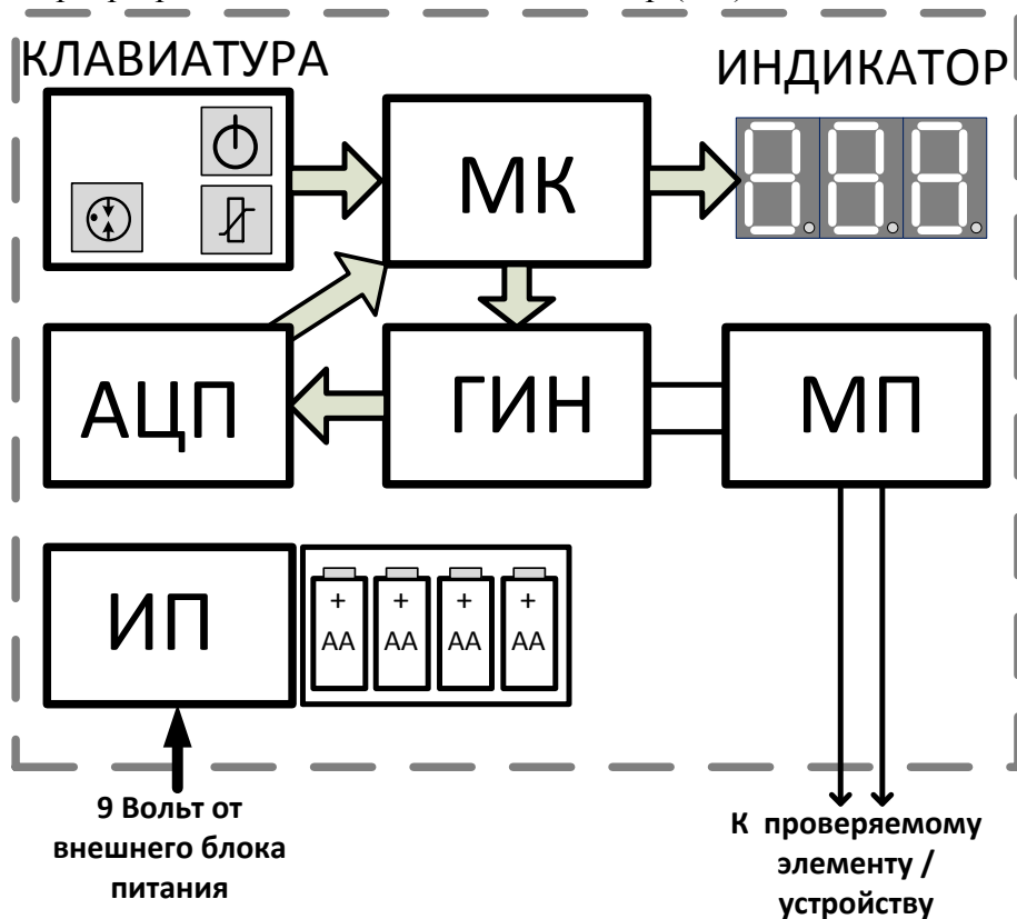
Рис. 1. Функциональная схема устройства «ISKRA»
