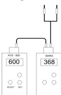
Рис. 3 Включение «ISKRA» и «AVS-800».
