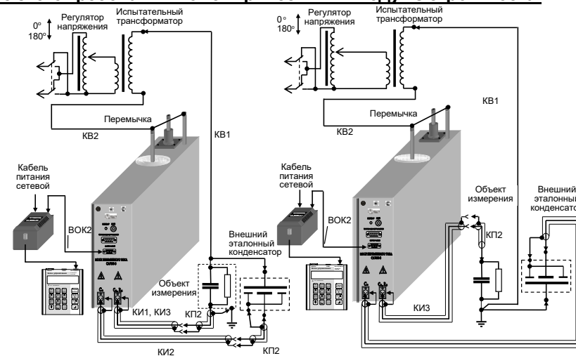
а – "прямая (нормальная)" схема б – "инверсная (перевернутая)" схема Рисунок 7.2
