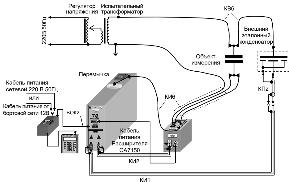
Схема измерительная при использовании внешнего эталонного конденсатора
