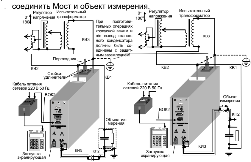
а – "прямая (нормальная)" схема б – "инверсная (перевернутая)" схема
