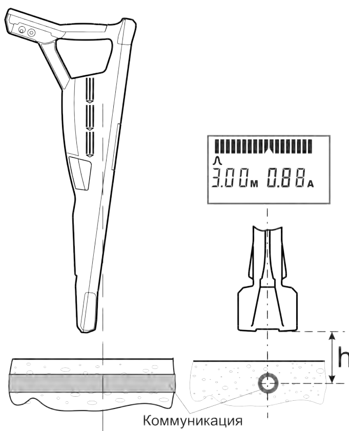
Рисунок 3.3.1 – Прямое определение глубины залегания
