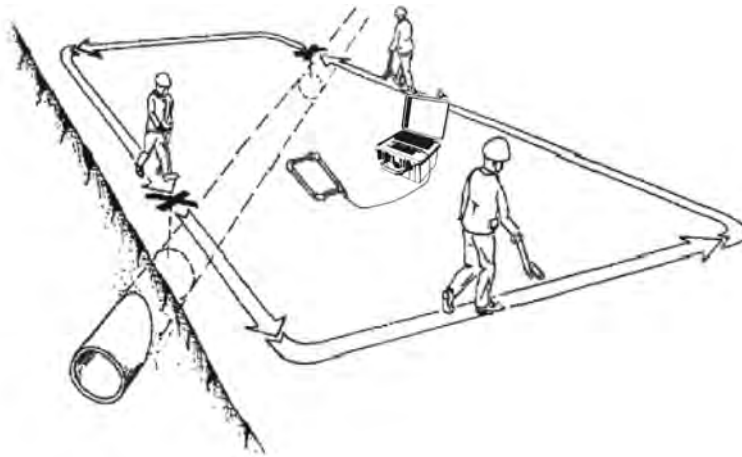
Рисунок 3.4.2.1 – Обследование участков местности с использованием рамки РП-02
